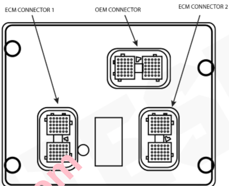
ECM CONNECTOR 2
