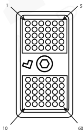
ECM CONNECTOR 2
